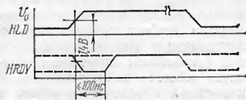
Рис. 4. Временные диаграммы сигналов загрузки и готовности МГ
